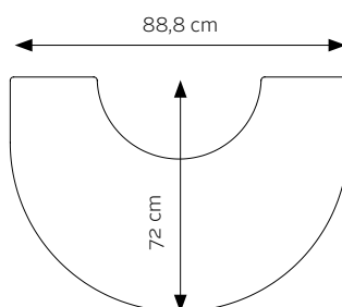
GULVPLADE TIL 7400 (PASSER IKKE TIL 7449) Varenr. 62929400
