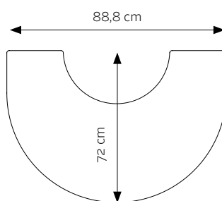
GULVPLADE TIL 7300 (PASSER IKKE TIL 7349) Varenr. 62929400
