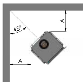
1446/1448 hjørnemontering
