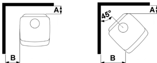
2140 hjørnemontering
