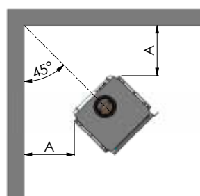
1446/1448 Eckmontage
