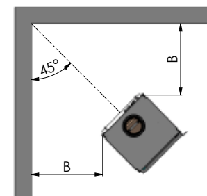
1416/1418 Eckmontage
