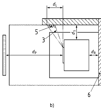
Sicherheitsabstände bei Verwendung eines isolierten Rauchrohrs und eines ungeschützten Rauchrohrstutzens
