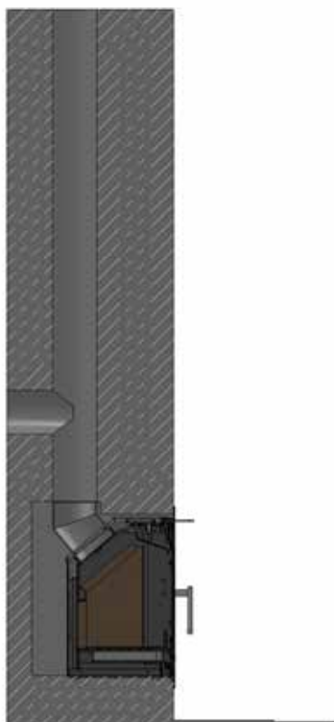
S81-go installeret i eksisterende murværk
